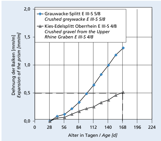
Bild 9: Dehnung von Betonen mit verschiedenen Gesteinskörnungen der Alkaliempfindlichkeitsklasse E III-S im 60 °C-Betonversuch mit Alkalizufuhr durch eine 3 %ige Natriumchloridlösung. CEM I 42,5 N, Na 2 O-Äquivalent = 0,62 M.-%, z = 430 kg/m 3 , w/z-Wert = 0,42, LP = 5,5 ± 0,5 Vol.-%, 30 Vol.-% Sand 0/2, 70 Vol.-% Grauwacke-Splitt E III-S 5/8 bzw. Kies-Edelsplitt E III-S 4/8
