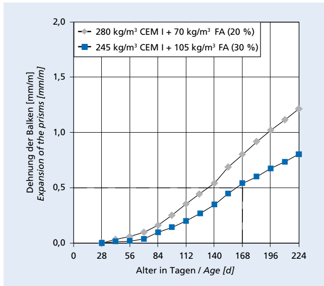
Bild 11: Dehnung von Betonen mit Grauwacke-Splitt der Alkaliempfindlichkeitsklasse E III-S, Portlandzement und Flugasche im 60 °C-Betonversuch mit Alkalizufuhr durch eine 3 %ige Natriumchloridlösung. CEM I 42,5 R, Na 2 O-Äqu. = 1,19 M.-%, z + f = 350 kg/m 3 , w/(z + f) = 0,45 (k = 1,0), 30 Vol.-% Sand 0/2, 70 Vol.-% Grauwacke E III-S 2/16 Figure 11: Expansion of concrete compositions made with crushed greywacke of the E III-S alkali reactivity class, Portland cement and fly ash in the 60 °C concrete test with external supply of alkalis through a 3 % sodium chloride solution. CEM I 42,5 cement, Na 2 O-equiv. = 1.19 mass %, c + f = 350 kg/m 3 , w/(c + f) = 0.45 (k = 1.0), 30 vol. % sand 0/2, 70 vol. % greywacke E III-S 2/16
